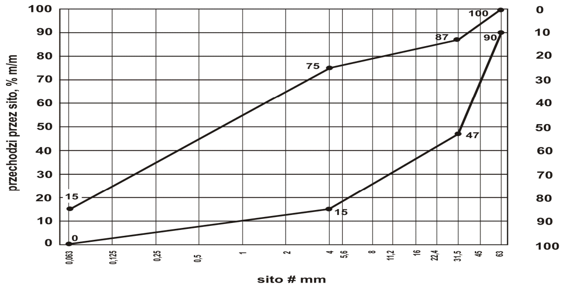
Rys. 5. Uziarnienie mieszanki niezwiązanej 0/63 dla nawierzchni
